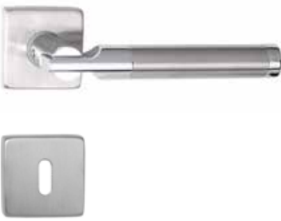
/// készleten RIMINI négyzetrozettás F fényes króm és szálcsiszolt acél A zamak és rozsdamentes acél M A=146 mm D=50 mm
