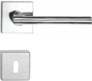
/// készleten DANIELA ECO F szálcsiszolt acél A rozsdamentes acél M A=126 mm D=50 mm
